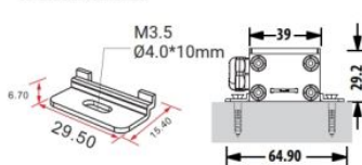
Montagehalter
